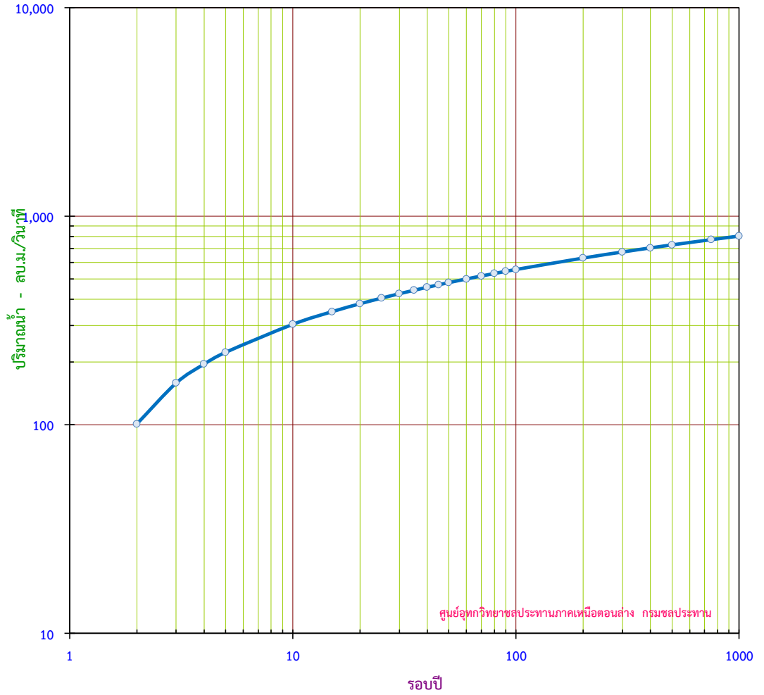
กราฟแสดง ปริมาณน้ำสูงสุดรายปี ขนาดรอบปีต่างๆ สถานี P.47 อ.คลองลาน จ.กำแพงเพชร
